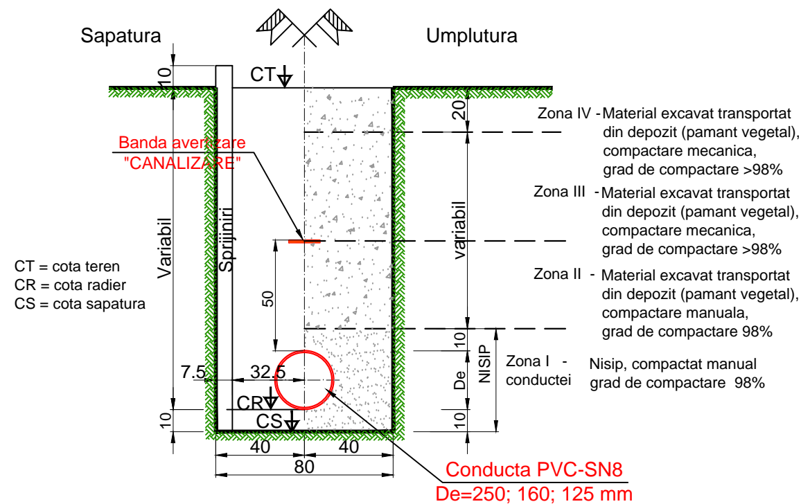
Detaliu pozare conducta gravitationala De= 250; 160; 125mm in zona verde
