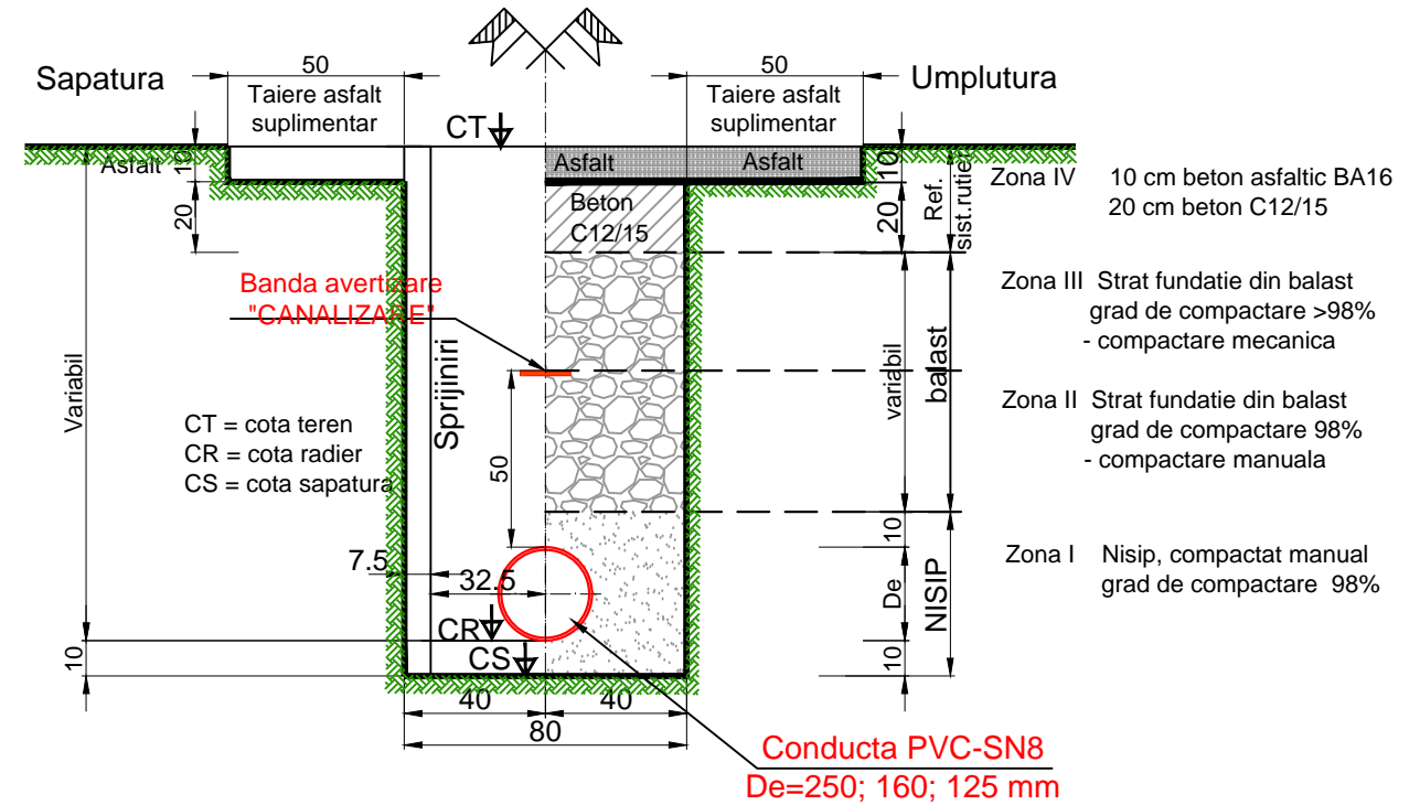
Detaliu pozare conducta gravitationala De=250;160; 125mm in zona drum asfaltat
